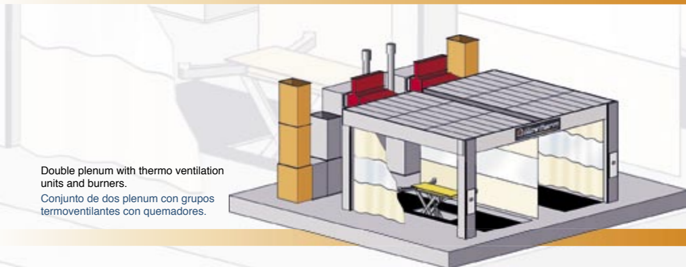
Double plenum with fitted storage walls. Conjunto de dos plenum con pared equipada.
